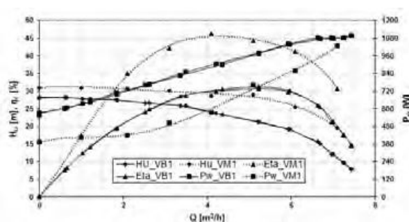
Rys. 10: Charakterystyka dla pompy z kanałem spiralnym
