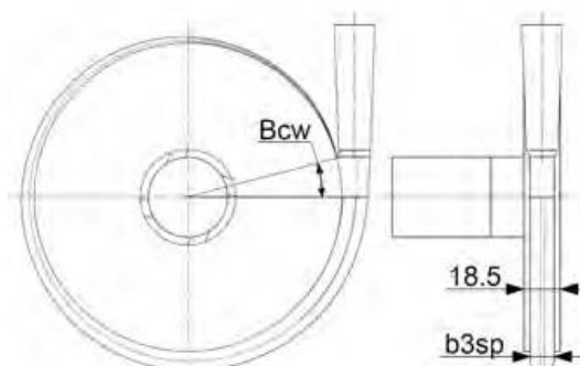
Rys. 8: Wymiary kanału spiralnego
